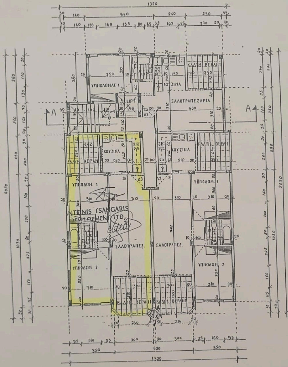
ΚΑΤΩΦΗ ΤΥΠΙΚΟΥ ΟΡΟΦΟΥ ( Β . Γ Δ )
