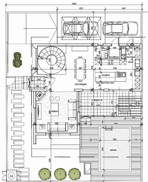
ΚΑΤΟΨΗ ΙΣΟΓΕΙΟΥ
