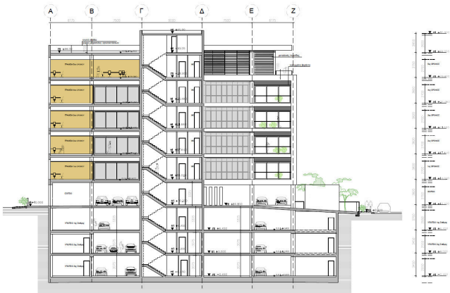
ТОМН B-B' 1:200
