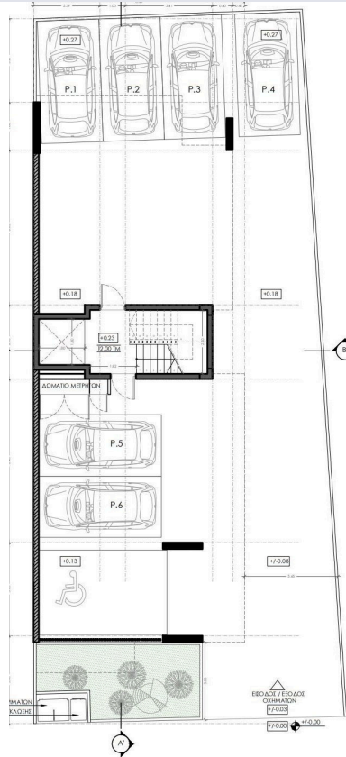
ΚΑΤΩΦΗ ΙΣΟΓΕΙΟΥ
